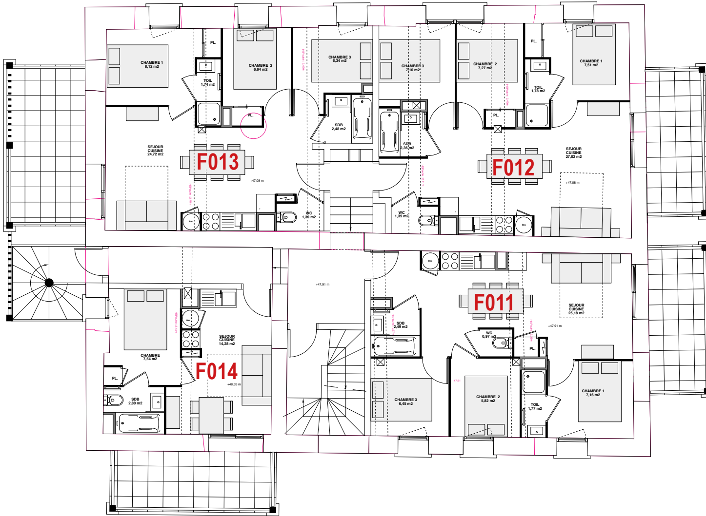
PLAN DU 1ER ETAGE - BATIMENT LA FREGATE
